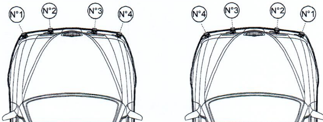
Posizione dei sensori nella vettura / Sensors position on the vehicle
